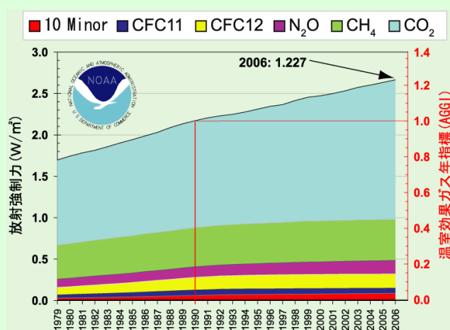
図2 長寿命の各温室効果ガスによる放射強制力の経年変化と2006 年の NOAA 温室効果ガス年指標(AGGI)。「10Minor」は、HCFC22、CFC113、CCl 4 などの10 種のアロゲンガスの合計
